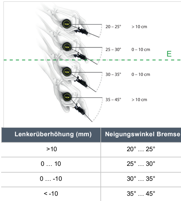
Abbildung 129: Neigungswinkel der Bremse
