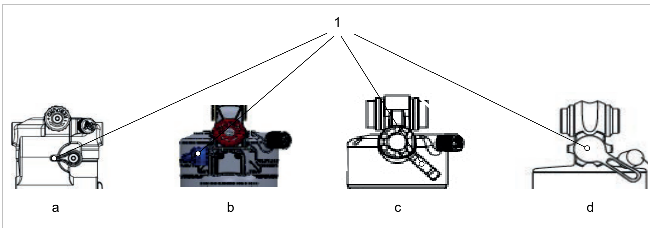
Abbildung 240: Lage RS Suntour Druckstufen-Hebel bei Hinterbau-Dämpfer Triair2 (a), Triair (b), EDGE-comp (c), EDGE (d)
