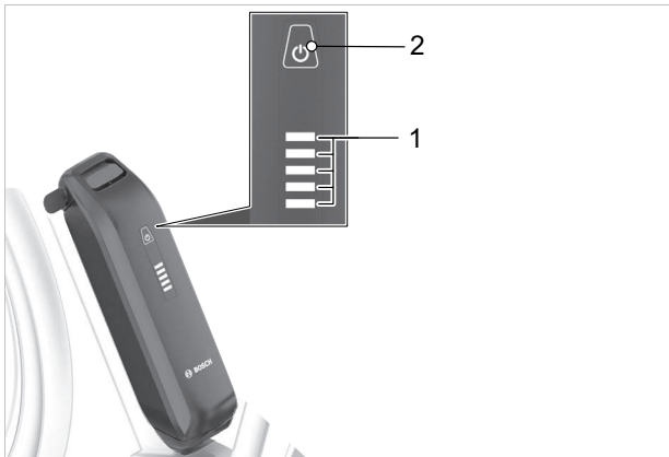
Abbildung 75: Anzeige und Bedienelement BOSCH PowerPack Akku
