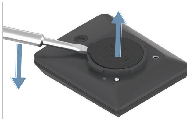
Abbildung 144: Batteriefach-Abdeckung hochheben
