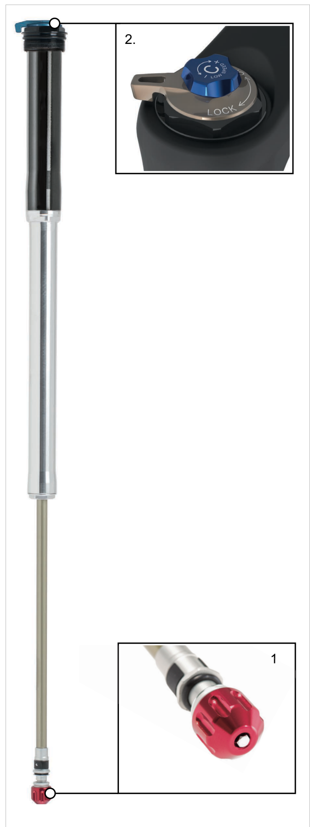
Abbildung 22: Bedienelemente des RL
