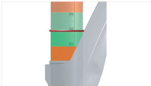
Abbildung 135: Vorgeschriebener SAG Bereich (grün) und verbotener AG Bereich (rot)
