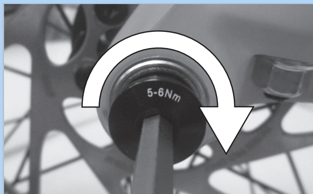
Abbildung 76: Sicherungsschraube anziehen
