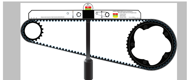
Abbildung 219: Lineal platziert
