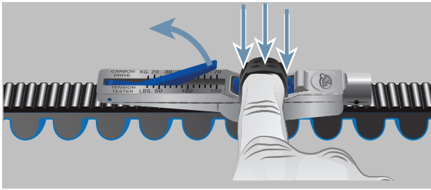
Abbildung 216: Prüfler mit Finger herunterdrücken
