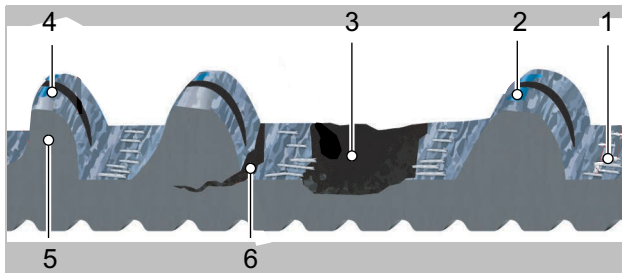
Abbildung 210: Verschleißmerkmale eines Riemens
