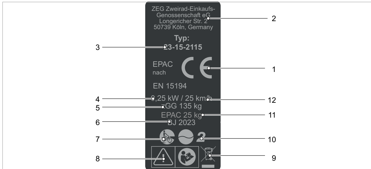
Abbildung 2: Beispiel Typenschild ZEG
