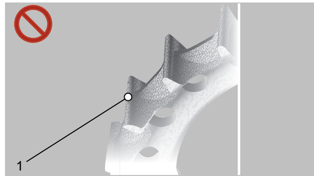
Abbildung 212: Verschlissenes Zahnprofil
