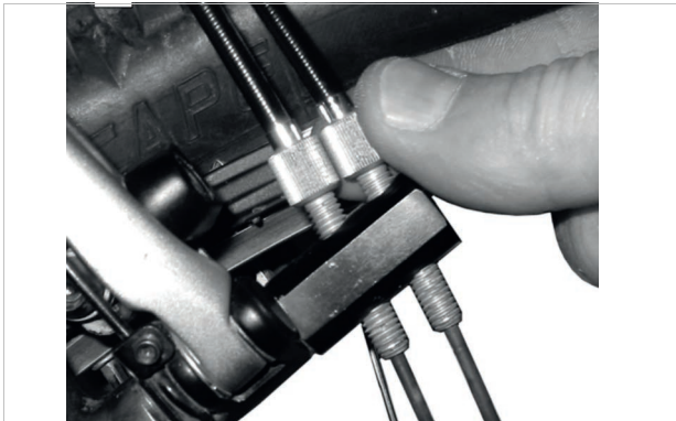
Abbildung 223: ROHLOFF-Naben Versionen mit interner Schaltansteuerung haben die Zugeinsteller am Zuggeghalter
