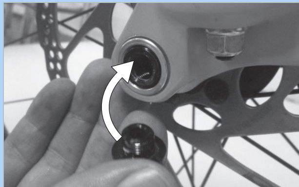
Abbildung 75: Sicherungsschraube einsetzen
