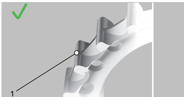
Abbildung 211: optimales Zahnprofil
