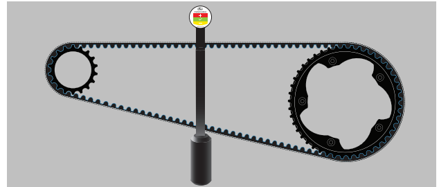
Abbildung 218: Aufgehängter Messstab
