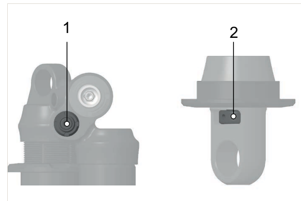
Abbildung 155: Lowspeed (1) und Highspeed (2) Zugstufe
