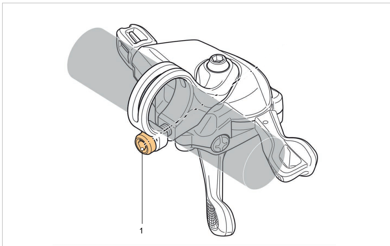
Abbildung 126: Lage Befestigungsschraube Schalthebel SHIMANO (1)
