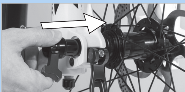
Abbildung 77: Querachse in Pfeilrichtung einschieben
