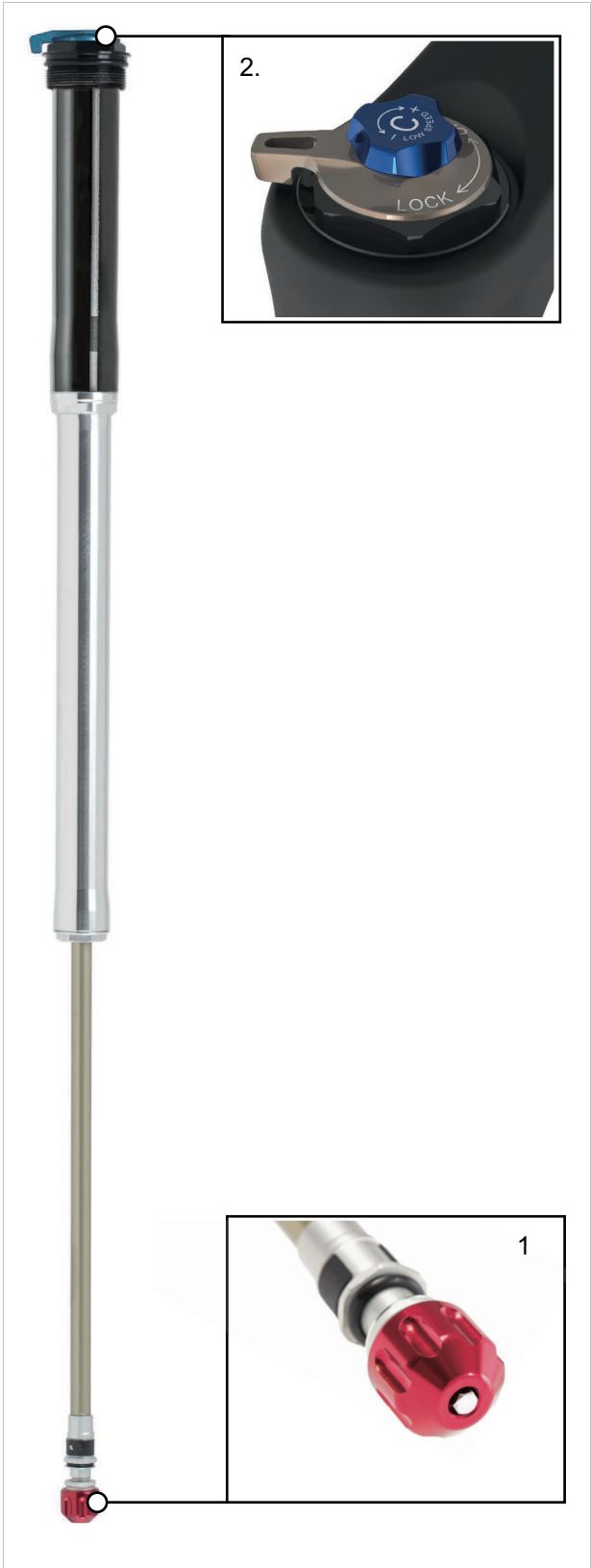
Abbildung 25: Bedienelemente des LOR
