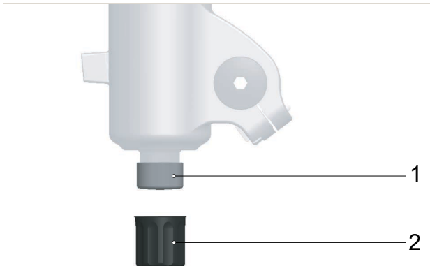
Abbildung 246: FOX Zugstufen-Einsteller (Gabel) (1) unter Gabel-Kappe (2)
