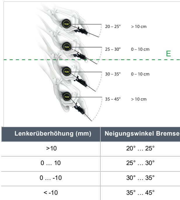
Abbildung 122: Neigungswinkel der Bremse
