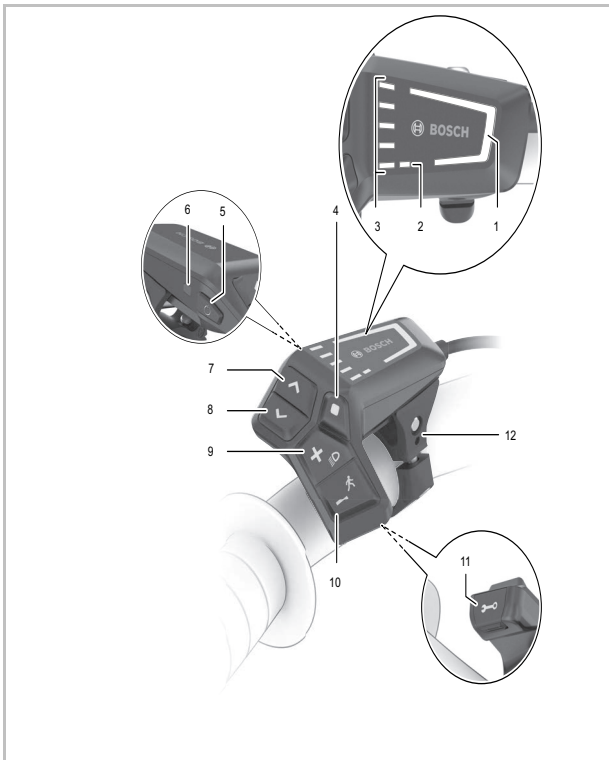
Abbildung 180: Übersicht Bedieneinheit BOSCH LCD Remote
