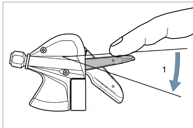
Abbildung 189: Schalten mit Hebel B, Beispiel Schaltung SL-M315
