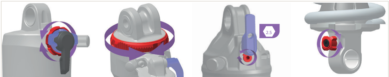
Abbildung 274: Lage und Form des Zugstufen-Einstellers (rot) ist Modellabhängig
