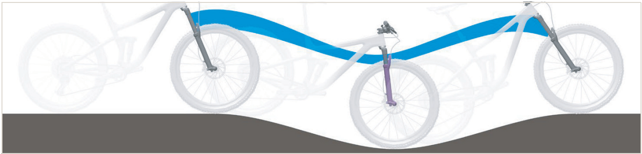
Abbildung 249: Zu weiche Federung der Federgabel am Berg
