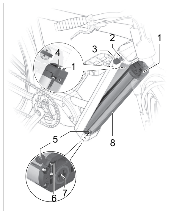
Abbildung 48: Details PowerTube
