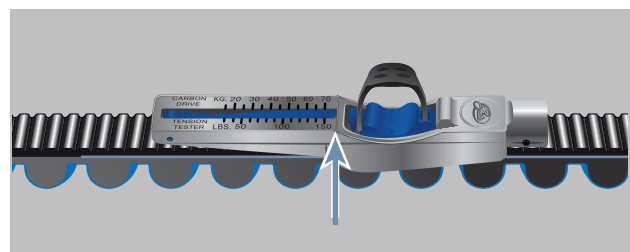
Abbildung 215: Prüflinse auf Riemen
