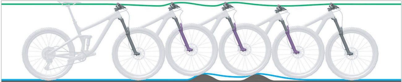
Abbildung 241: Zu langsames Ausfedern der Federgabel
