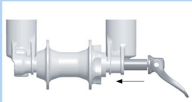
Abbildung 87: Schnellspanner einschieben
