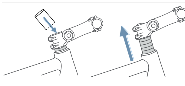
Abbildung 114: Ahead-Vorbau durch Einbau von Distanzringe (Spacer) erhöhen
