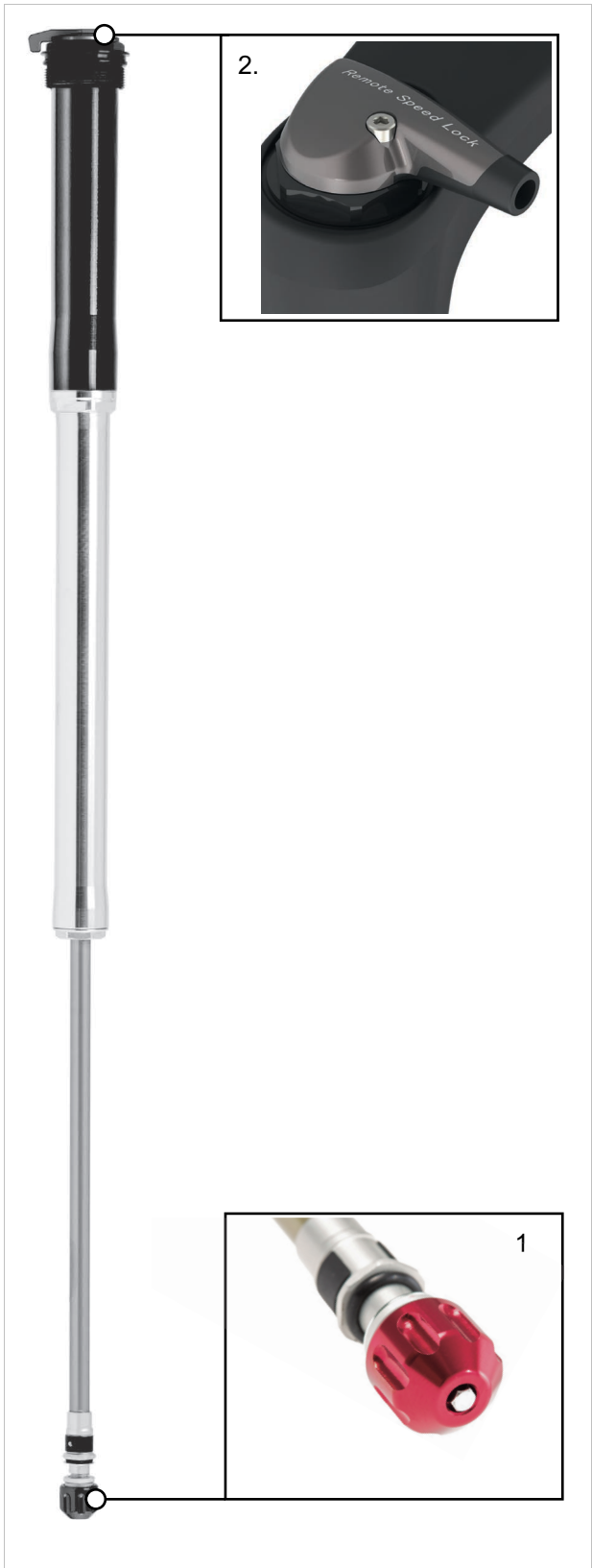
Abbildung 28: Bedienelemente der RLR Kartusche
