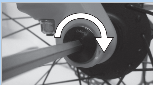
Abbildung 74: Achse in Pfeilrichtung anziehen
