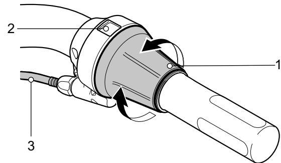
Abbildung 45: Schaltung SHIMANO SL-C30000-7O
