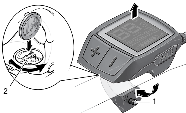
Abbildung 130: Bordcomputer mit Befestigungsschraube (1) und Batteriefachdeckel (2)
