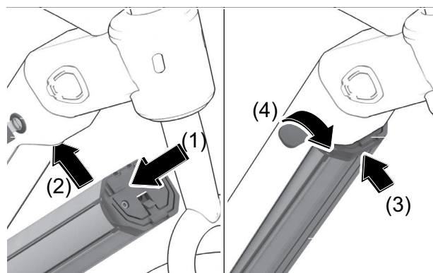
Abbildung 127: Integrierten Akku einsetzen
