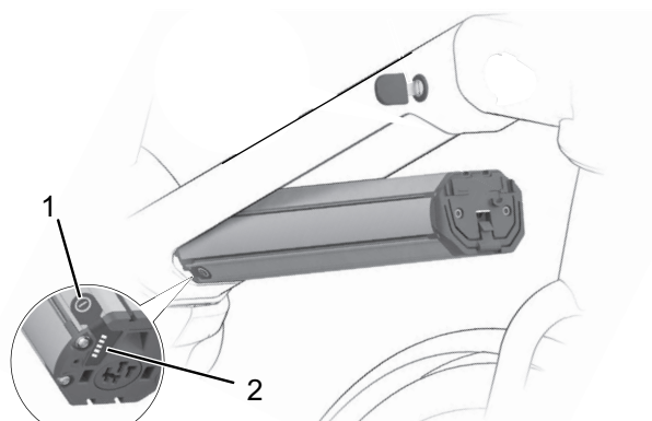
Abbildung 49: Lage Ladezustandsanzeige integrierter Akku
