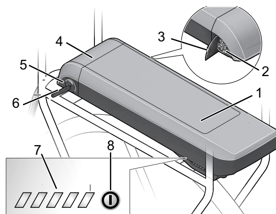
Abbildung 35: Detail Gepäckträgerakku
