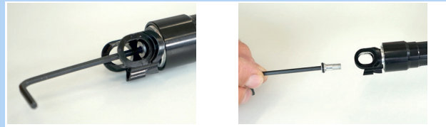
Abbildung 177: Ventilkappe herausdrehen
