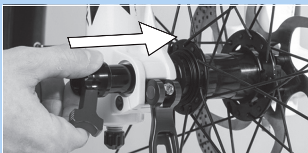
Abbildung 69: Querachse in Pfeilrichtung einschieben
