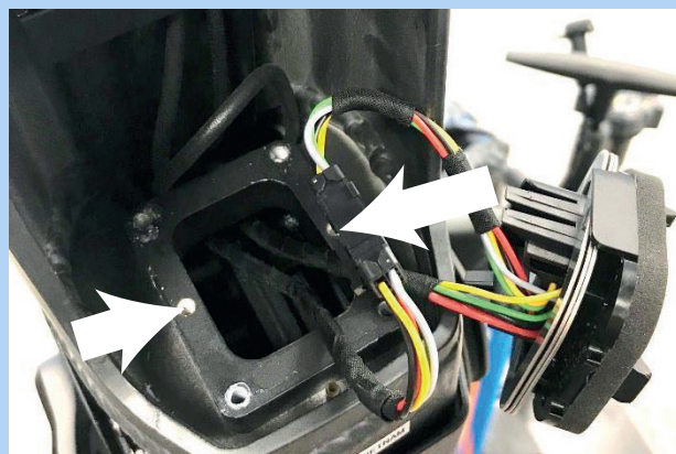
Abbildung 57: Akkuhalter festziehen
