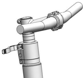
Abbildung 137: Beispiel All Up mit geöffnetem Vorbau-Spannhebel
