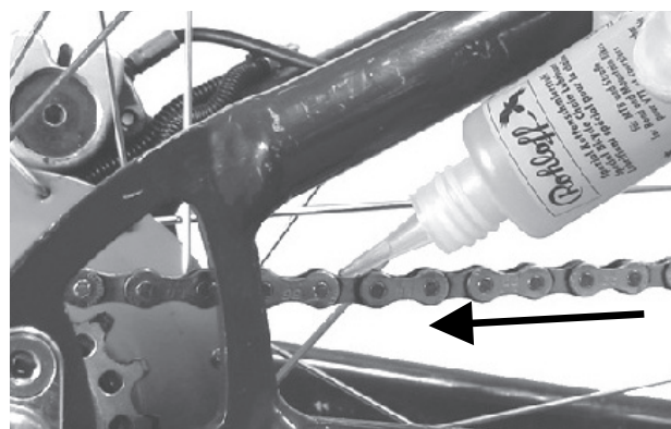
Abbildung 141: Kette schmieren
