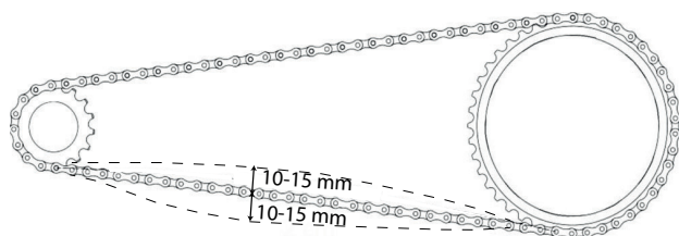
Abbildung 148: Kettenspannung prüfen
