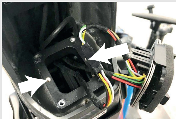
Abbildung 30: Akkuhalter festziehen
