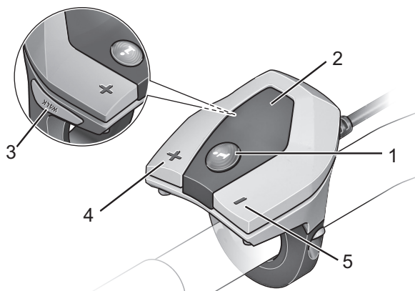
Abbildung 21: Übersicht Bedienteil
