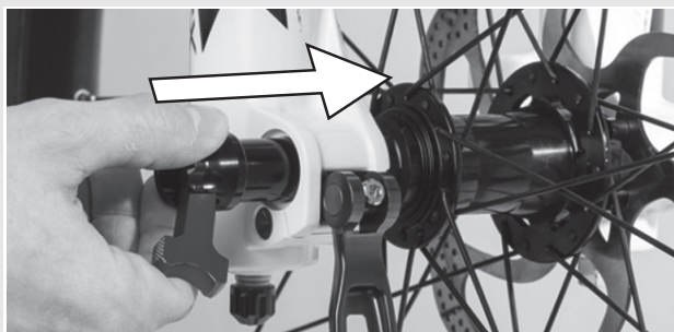
Abbildung 37: Achse in Nabe schieben
