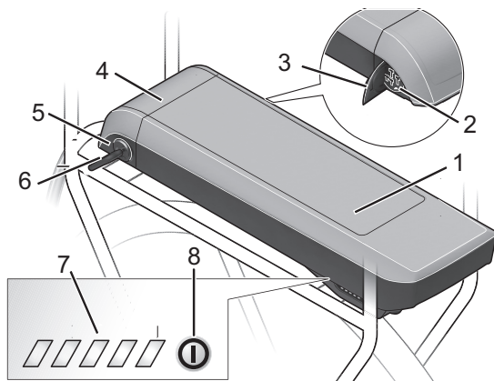
Abbildung 13: Detail Gepäckträgerakku
