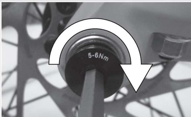
Abbildung 34: Sicherungsschraube anziehen
