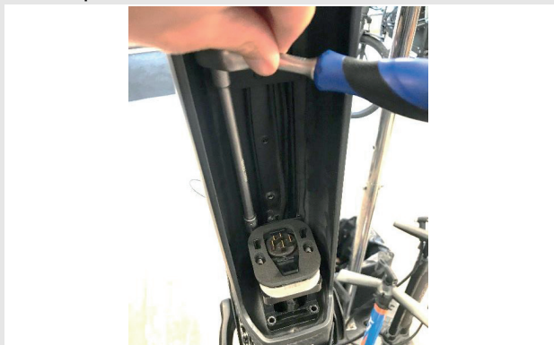
Abbildung 27: Innensechskant-Schrauben entfernen
