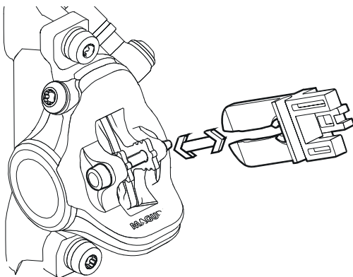
Abbildung 24: Transportsicherung befestigen
