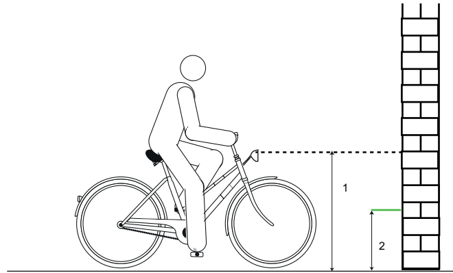
Abbildung 155: Frontleuchtehöhe (1) und die halbe Scheinwerferhöhe (2)
