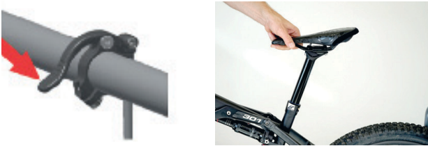
Abbildung 95: Hydraulische Gasdruckfeder ausfahren
