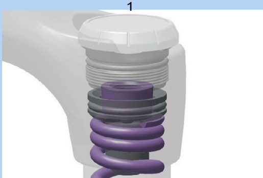
Abbildung 131: Vorspannungseinstellring hinein und heraus drehen.
