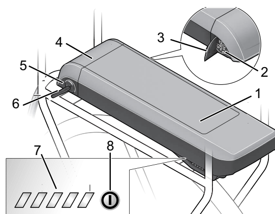
Abbildung 41: Detail Gepäckträgerakku
