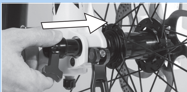
Abbildung 75: Querachse in Pfeilrichtung einschieben
