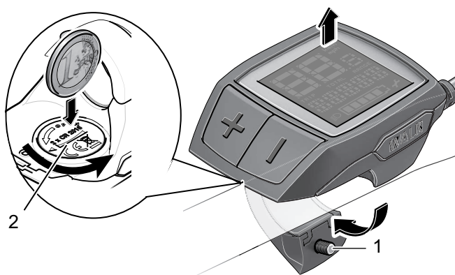
Abbildung 171: Bordcomputer mit Befestigungsschraube (1) und Batteriefachdeckel (2)
