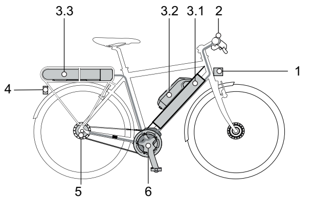
Abbildung 36: Schema elektrisches Antriebssystem mit elektrischen Bauteilen
