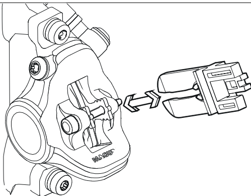
Abbildung 54: Transportsicherung befestigen
