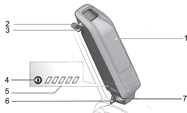
Abbildung 38: Detail Rahmenakku
