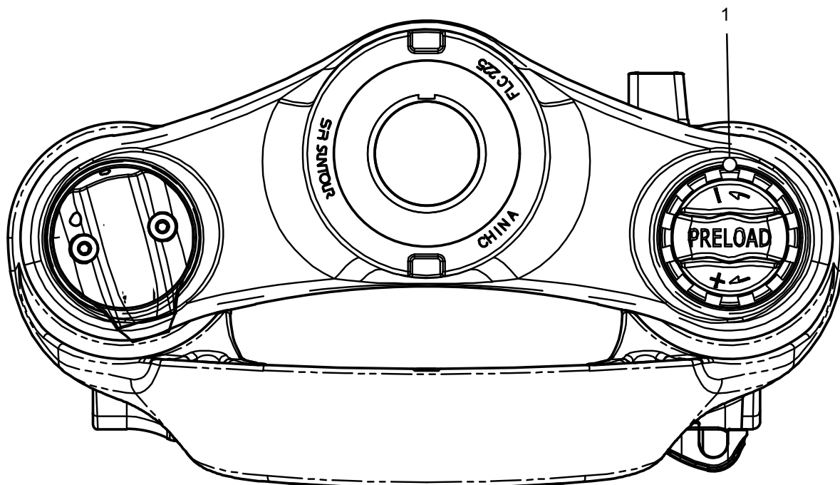
Abbildung 113: Einstellrad SAG (1) auf der Krone der Federgabel
