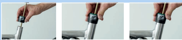
Abbildung 205: Außenhülse aufstecken
