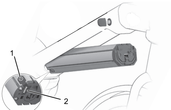
Abbildung 52: Lage Ladezustandsanzeige integrierter Akku
