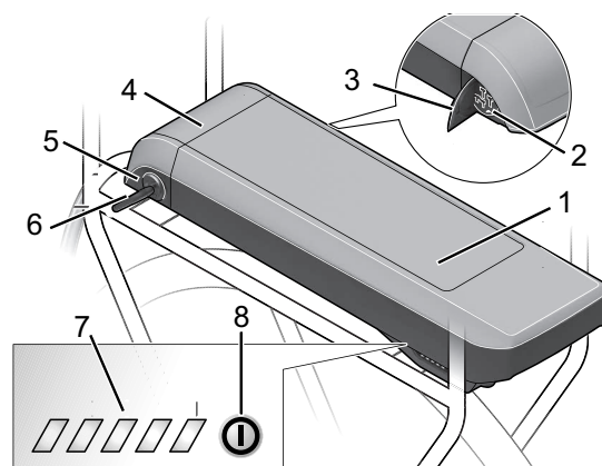
Abbildung 40: Detail Gepäckträgerakku
