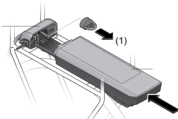
Abbildung 137: Offene Kontakte mit Abdeckklappe abdecken, Beispiel Gepäckträger
