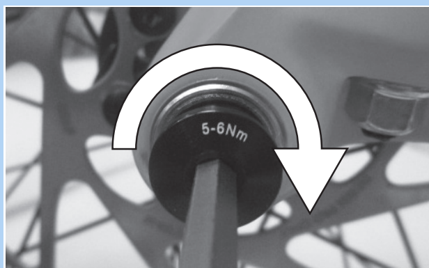
Abbildung 73: Sicherungsschraube anziehen
