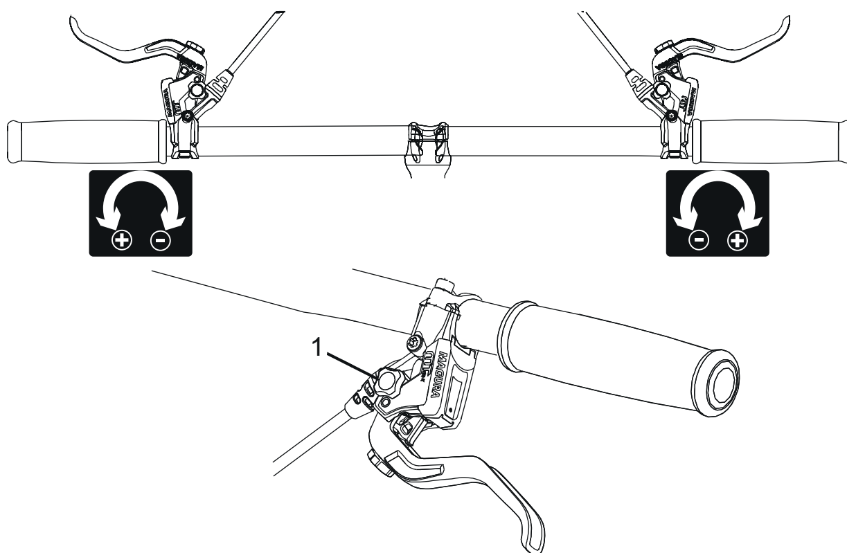
Abbildung 110: Benutzung des Drehknopfs (1) zur Druckpunkt-Einstellung
