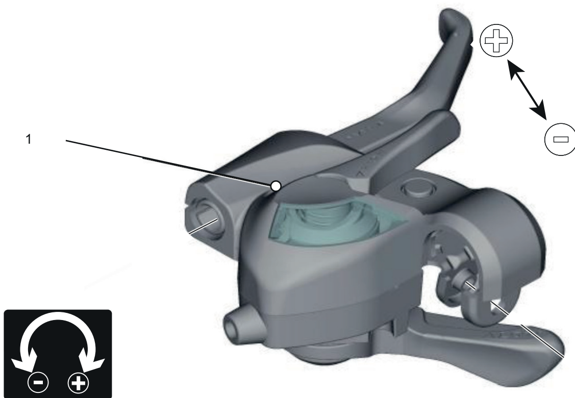
Abbildung 112: Lage Stellschraube (1)
