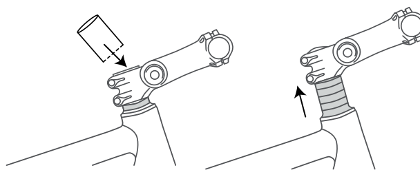
Abbildung 101: Ahead-Vorbau durch Einbau von Distanzringe (Spacer) erhöhen
