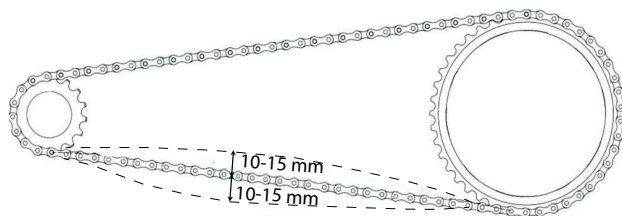
Abbildung 165: Kettenspannung prüfen
