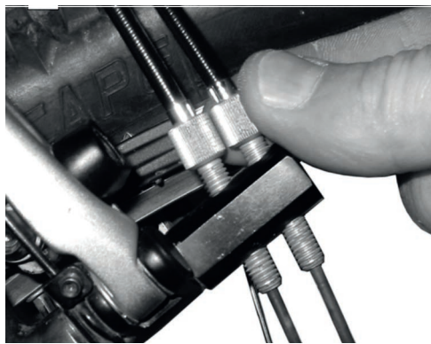
Abbildung 166: ROHLOFF-Naben Versionen mit interner Schaltansteuerung haben die Zugeinsteller am Zuggegenhalter
