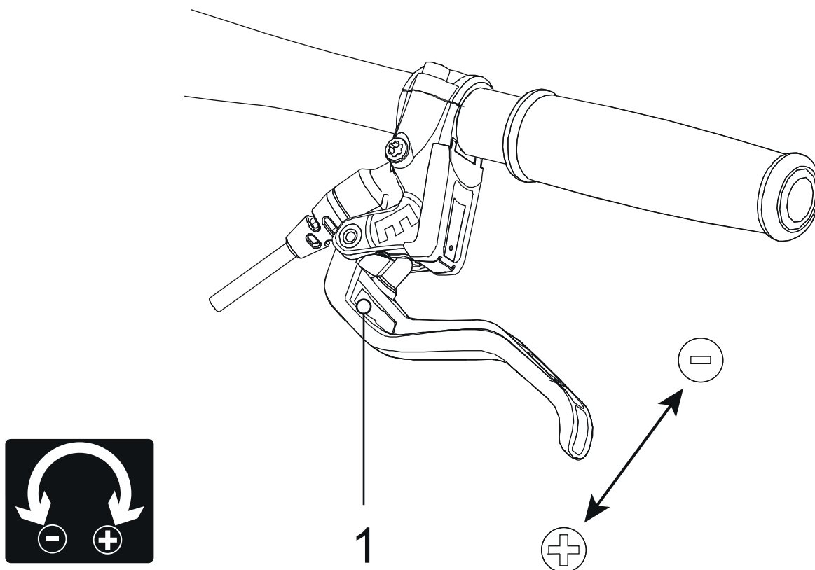
Abbildung 108: Griffweite Bremshebel MAGURA HS 33 einstellen
