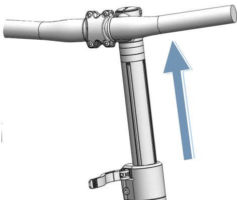
Abbildung 129: Beispiel All Up auf höchste Position gezogen
