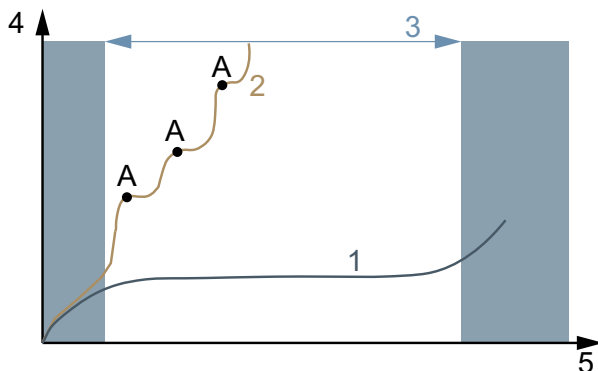
Abbildung 157: Diagramm Verschleiß, Betriebsdauer (x) zu Werstoffabtrag (y)
