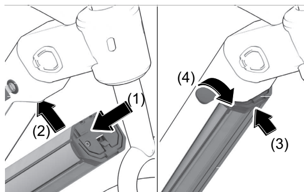
Abbildung 136: Integrierten Akku einsetzen
