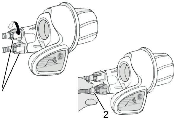
Abbildung 169: Drehgriffschalter mit Einstellhülsen (1) und Spiel der Gangschaltung (2)
