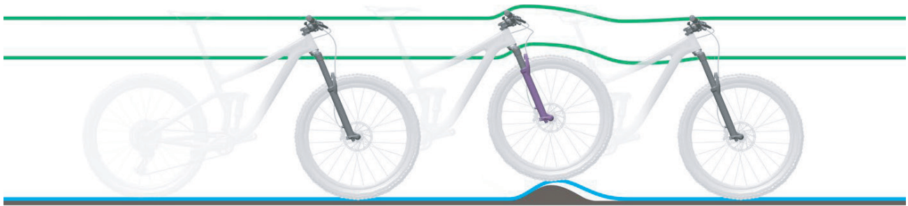
Abbildung 241: Zu harte Dämpfung der Federgabel bei Unebenheiten
