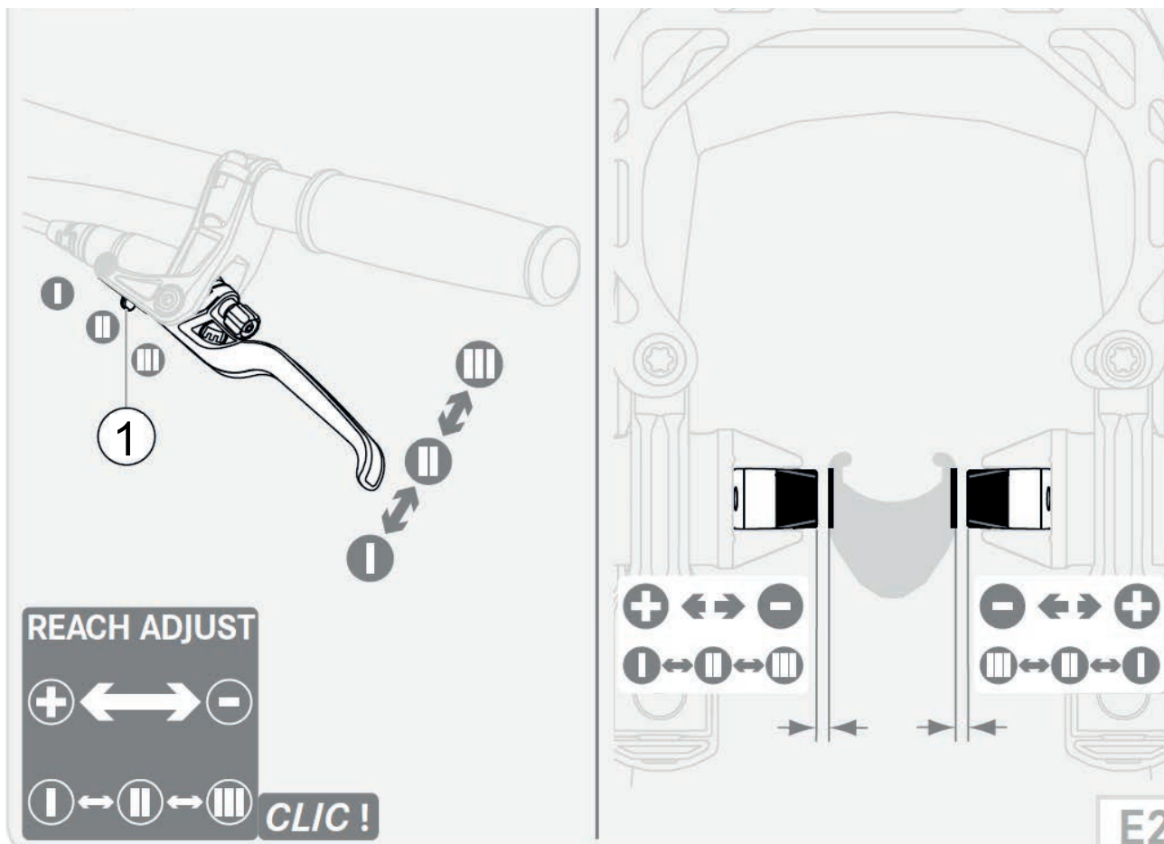
Abbildung 107: Griffweite Bremshebel MAGURA HS 22 einstellen
