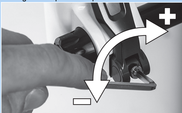
Abbildung 171: Spannkraft des Schnellspanners einstellen
