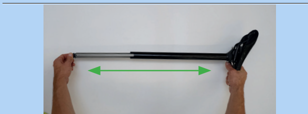
Abbildung 225: Sattelstütze auseinander ziehen
