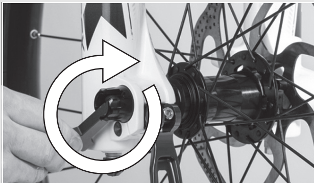
Abbildung 35: Achse anziehen
