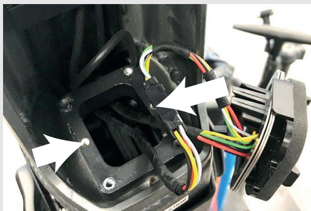
Abbildung 27: Akkuhalter festziehen
