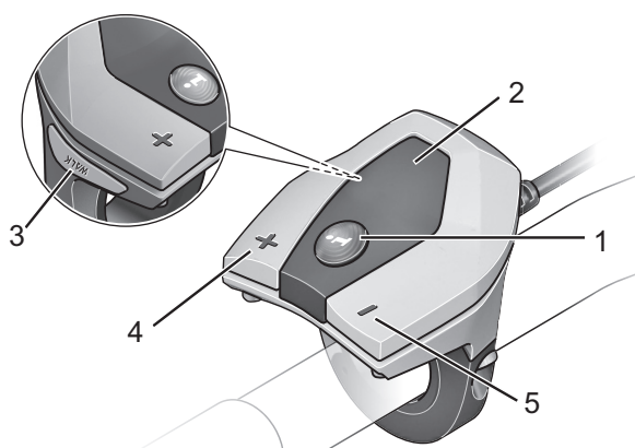
Abbildung 19: Übersicht Bedienteil
