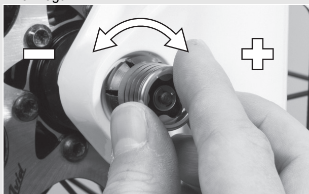
Abbildung 42: Spannung einstellen
