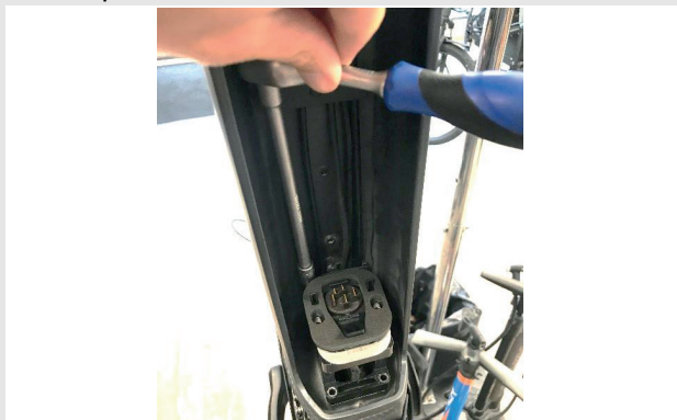
Abbildung 24: Innensechskant-Schrauben entfernen
