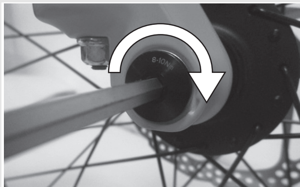
Abbildung 29: Achse anziehen
