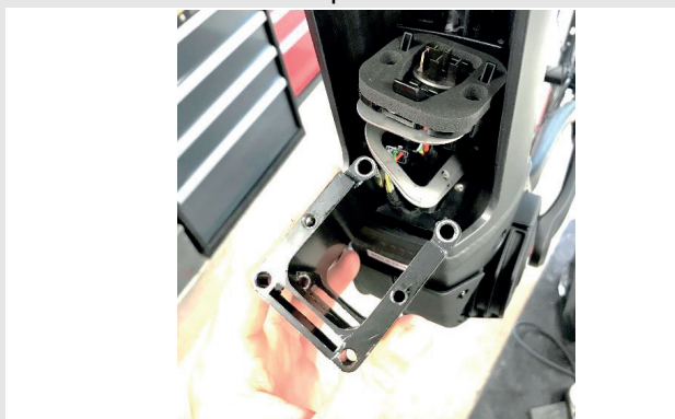
Abbildung 25: PowerTube Adapter herausziehen
