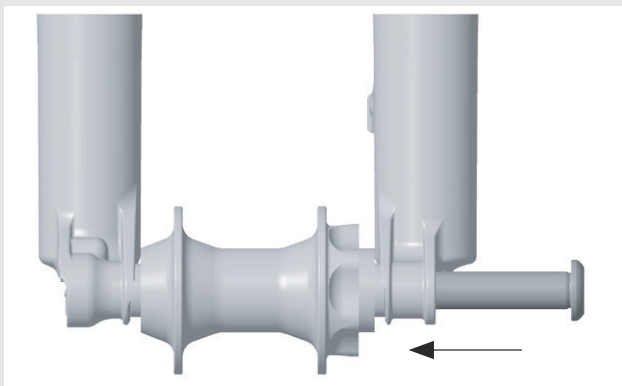
Abbildung 47: Kabolt-Achse einschieben
