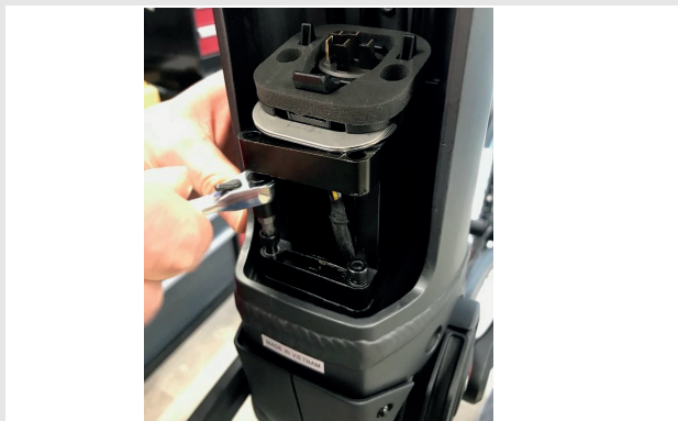
Abbildung 23: 4 mm 6-Kant-Schrauben entfernen
