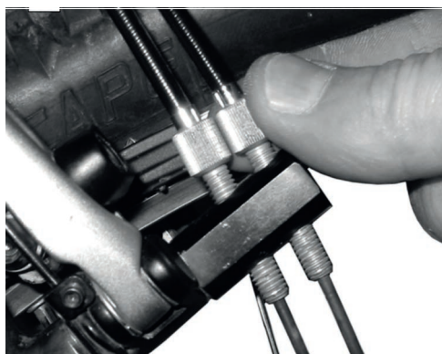
Abbildung 167: ROHLOFF-Naben Versionen mit interner Schaltansteuerung haben die Zugeinsteller am Zuggegenhalter
