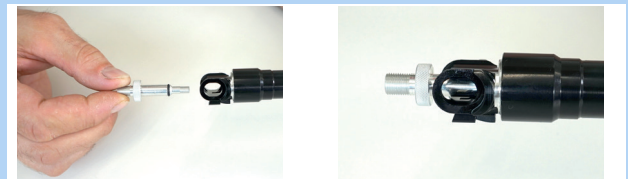
Abbildung 191: Ventiladapter einschrauben
