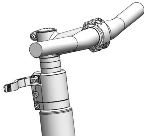
Abbildung 155: All Up mit geöffnetem Vorbau-Spannhebel
