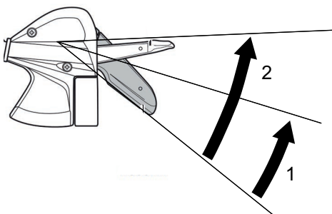
Abbildung 153: Schalten mit Hebel A, Beispiel Schaltung SL-M315
