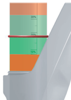
Abbildung 100: Vorgeschriebener SAG Bereich (grün) und verbotener SAG Bereich (rot)
