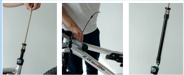
Abbildung 178: Kartusche herausziehen
