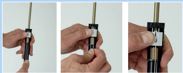
Abbildung 179: Seilzug aushängen
