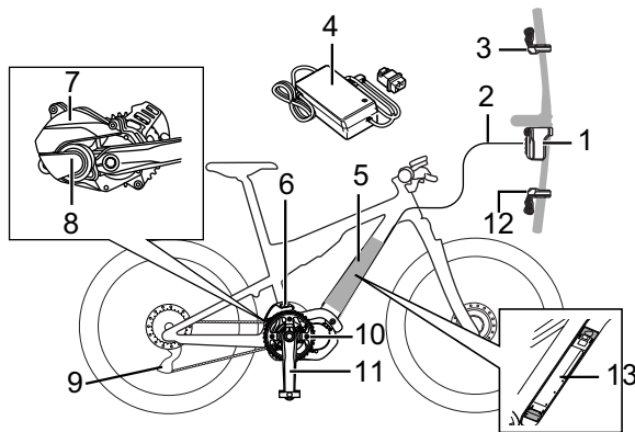
Abbildung 39: Schema Elektrisches Antriebssystem
