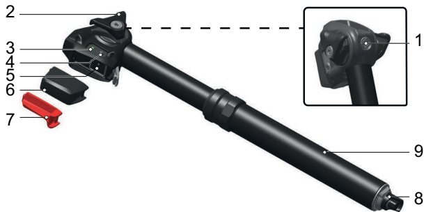
Abbildung 34: Aufbau ROCKSHOX Reverb AXS Sattelstütze
