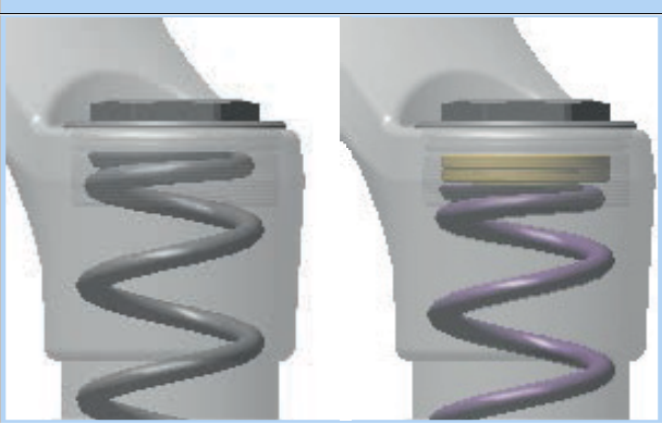
Abbildung 92: Vorspannungseinstellring hinein und heraus drehen.
