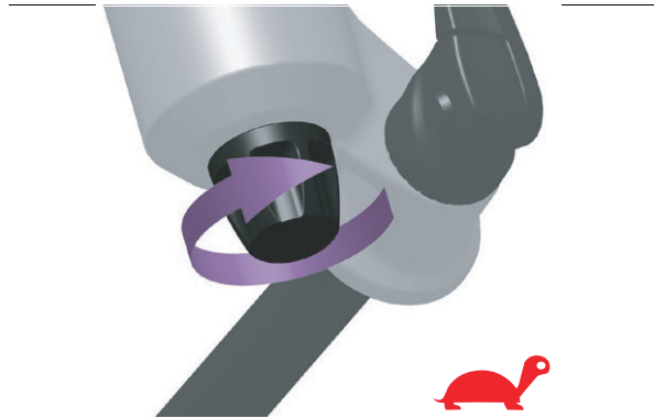
Abbildung 237: Zugstufen-Schraube in Richtung Schildkröte drehen
