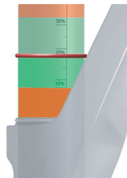
Abbildung 91: Vorgeschriebener SAG Bereich (grün) und verbotener SAG Bereich (rot)
