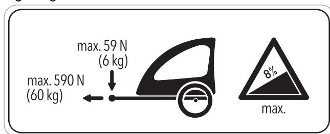
Hinweisschild Anhänger
