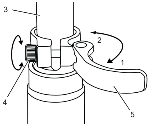
Abbildung 33: Schnellspanner der Sattelstütze (3) mit Spannhebel (5) und Einstellschraube (4) in geöffneter Position (1) und die Richtung der geschlossenen Position (2)
